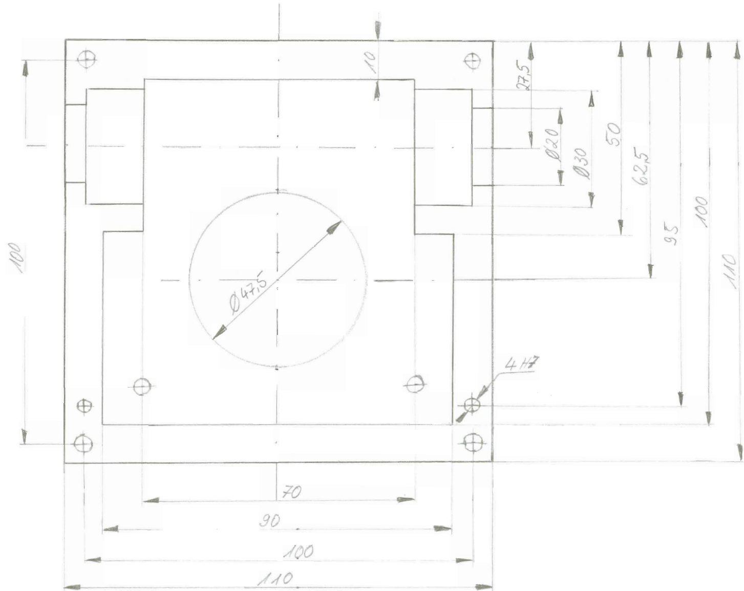
Gehäuse deckel
